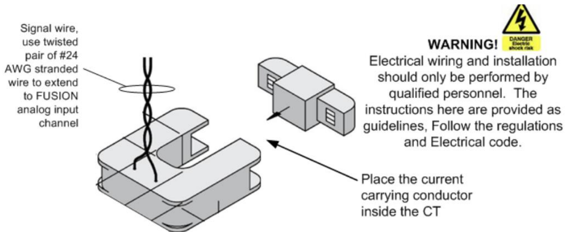
Figure 17 : Mesures de courant CA monophasé
