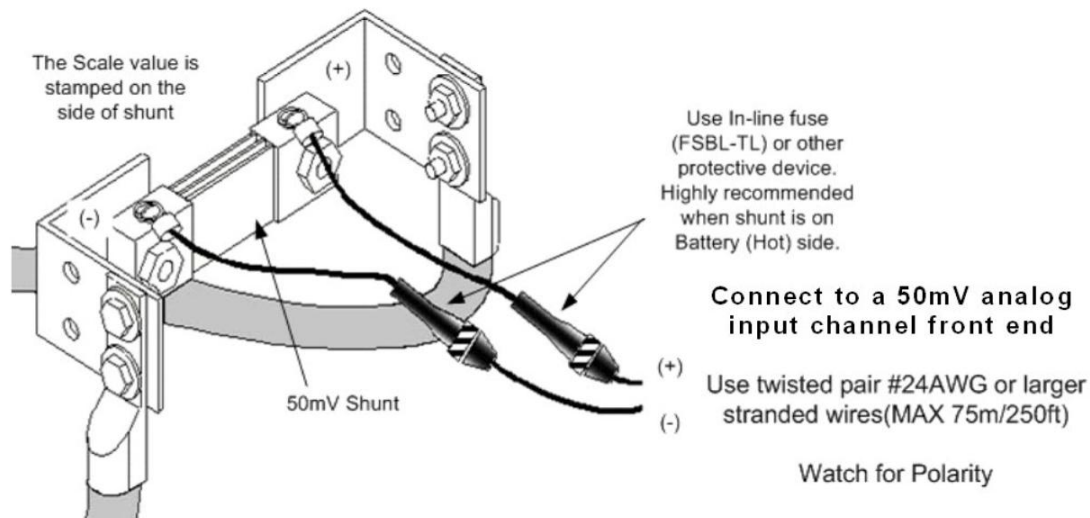
Figure 10 : Mesure de shunt CC
