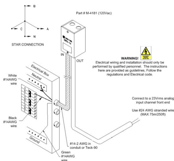
Figure 18 : Mesure monophasée 120 volts
