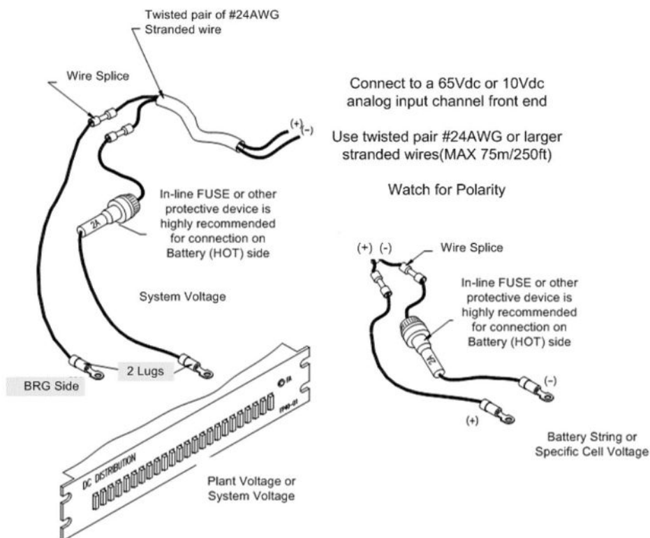
Figure 9 : Mesure de tension CC
