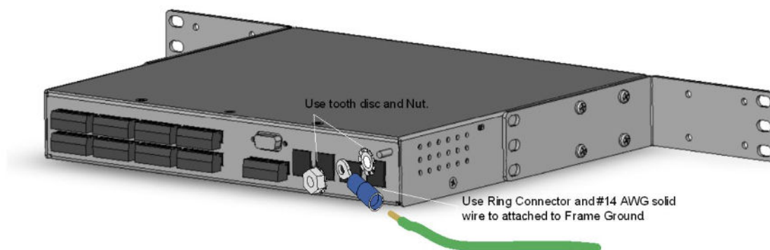
Figure 4 : Câblage de mise à la terre du châssis – entrée d'alimentation
