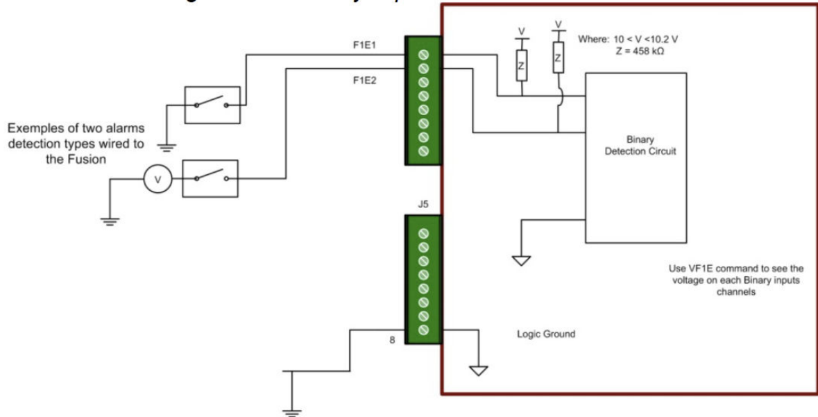
Figure 20 : Circuit de détection des canaux d'entrée binaire
