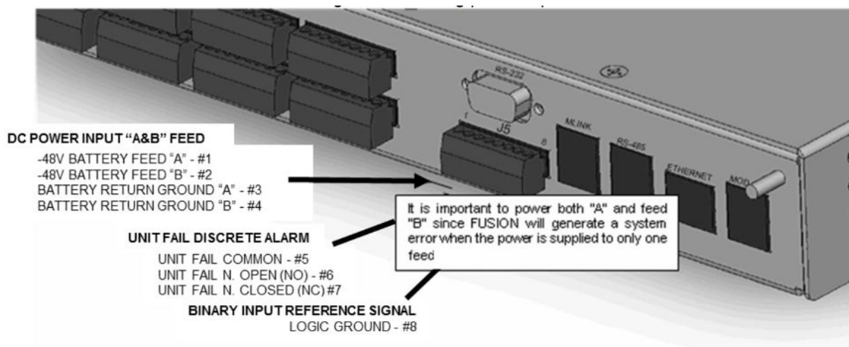
Figure 5 : Câblage de l'entrée d'alimentation
