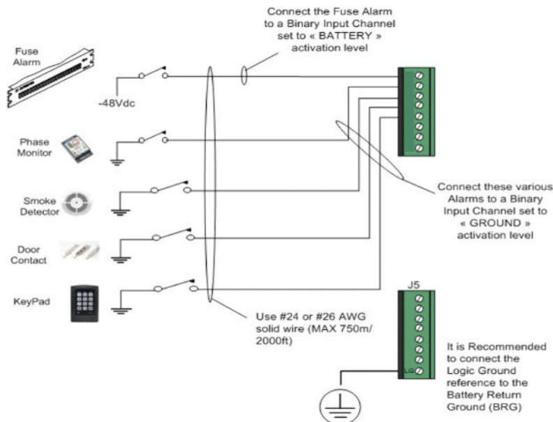
Figure 21 : Connexions des canaux d'entrée binaire
