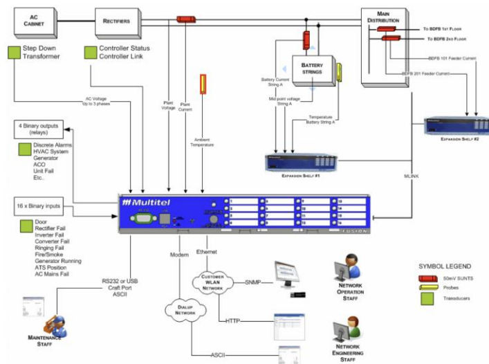
Figure 1 : Application typique de surveillance d'infrastructure
