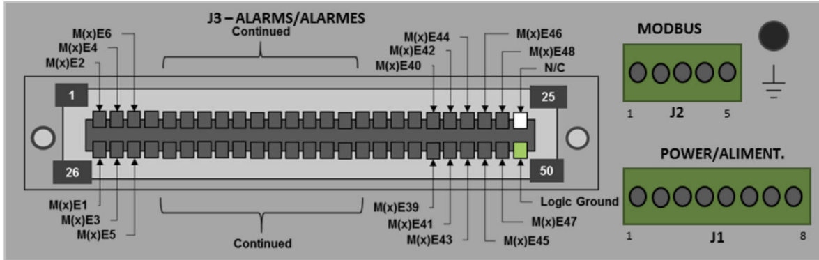
Figure 7 : Brochage des canaux d'entrée binaire du SMX-48BI
